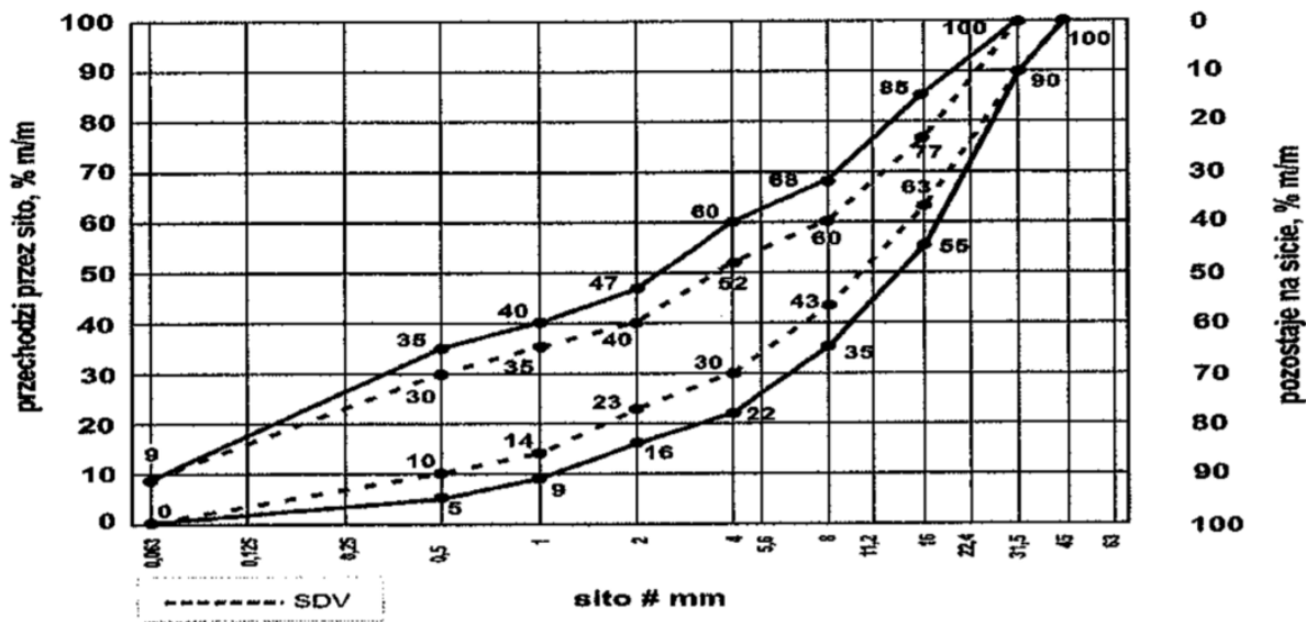
Rys. A. Pole dobrego uziarnienia dla mieszanki z kruszywa łamanego 0/31,5 do warstwy podbudowy zasadniczej wg WT-4
